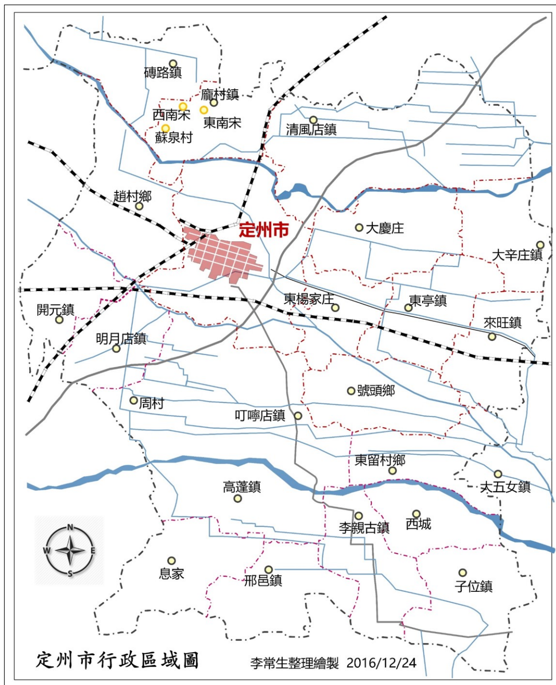
圖 19004：定州市行政區域圖。
