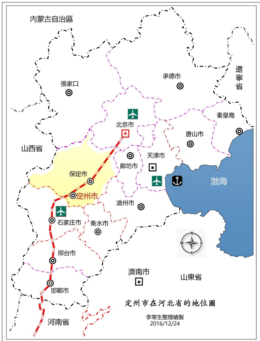
圖 19002：定州市在河北省的地位。
