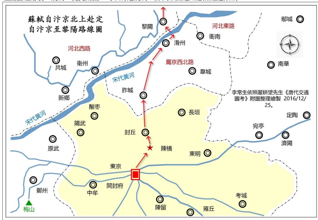
圖19014：蘇軾自汴京北上赴定自汴京至黎陽路線圖 1 。
