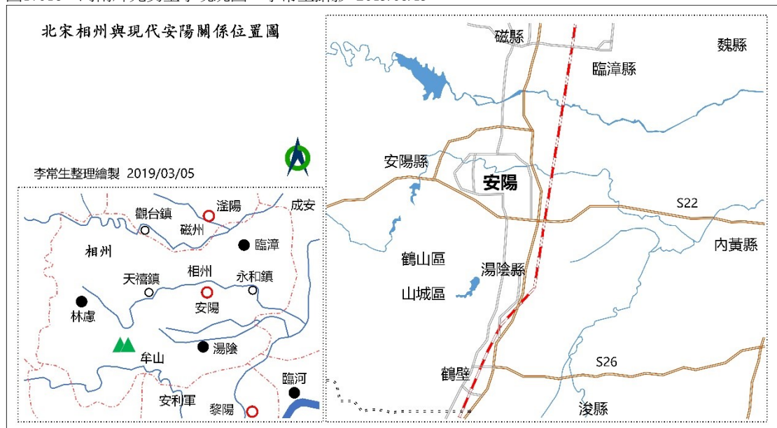
圖17019：北宋相州與現代安陽關係位置圖 2 。
