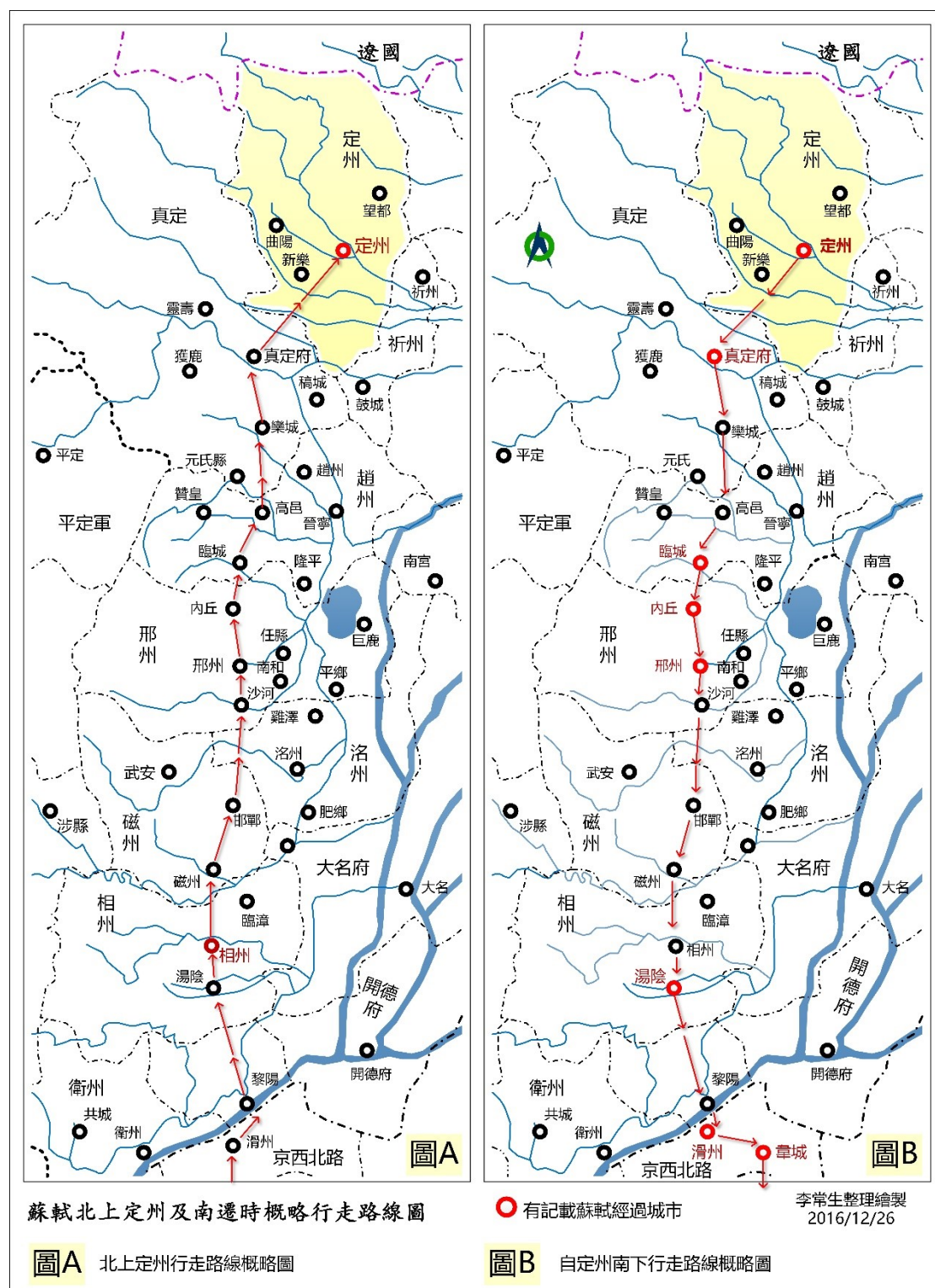
圖 19015：蘇軾北上定州及南遷時行走路線圖 1 。
