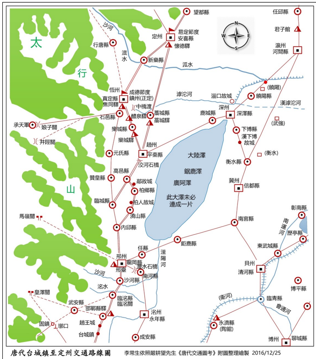
圖19012：唐代台城鎮至定州交通路線圖 1 。說明：汴京往北至定州，主要路線經過樂城驛、樂城縣。
