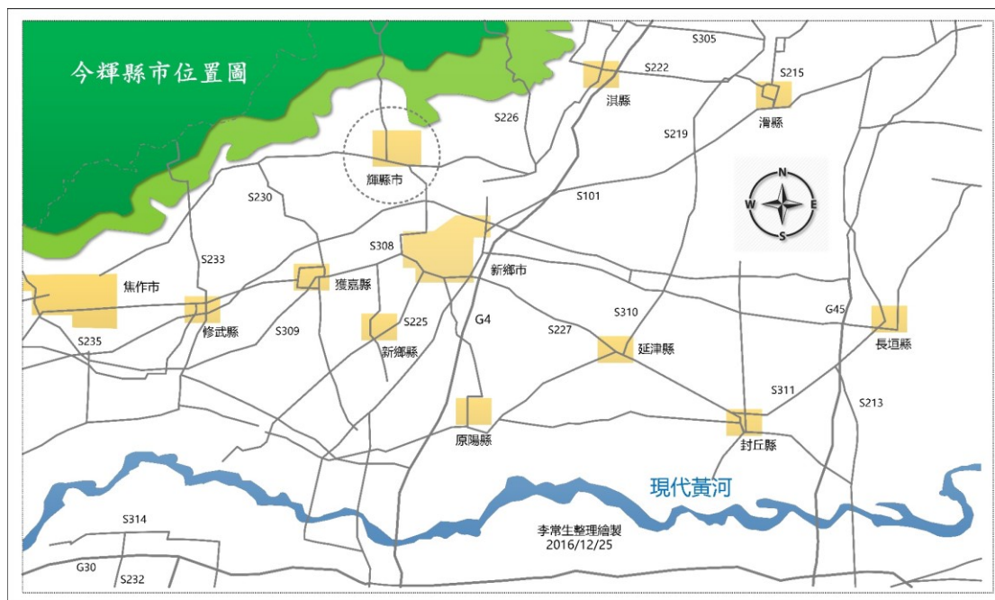
圖 17016：今輝縣位置圖。
